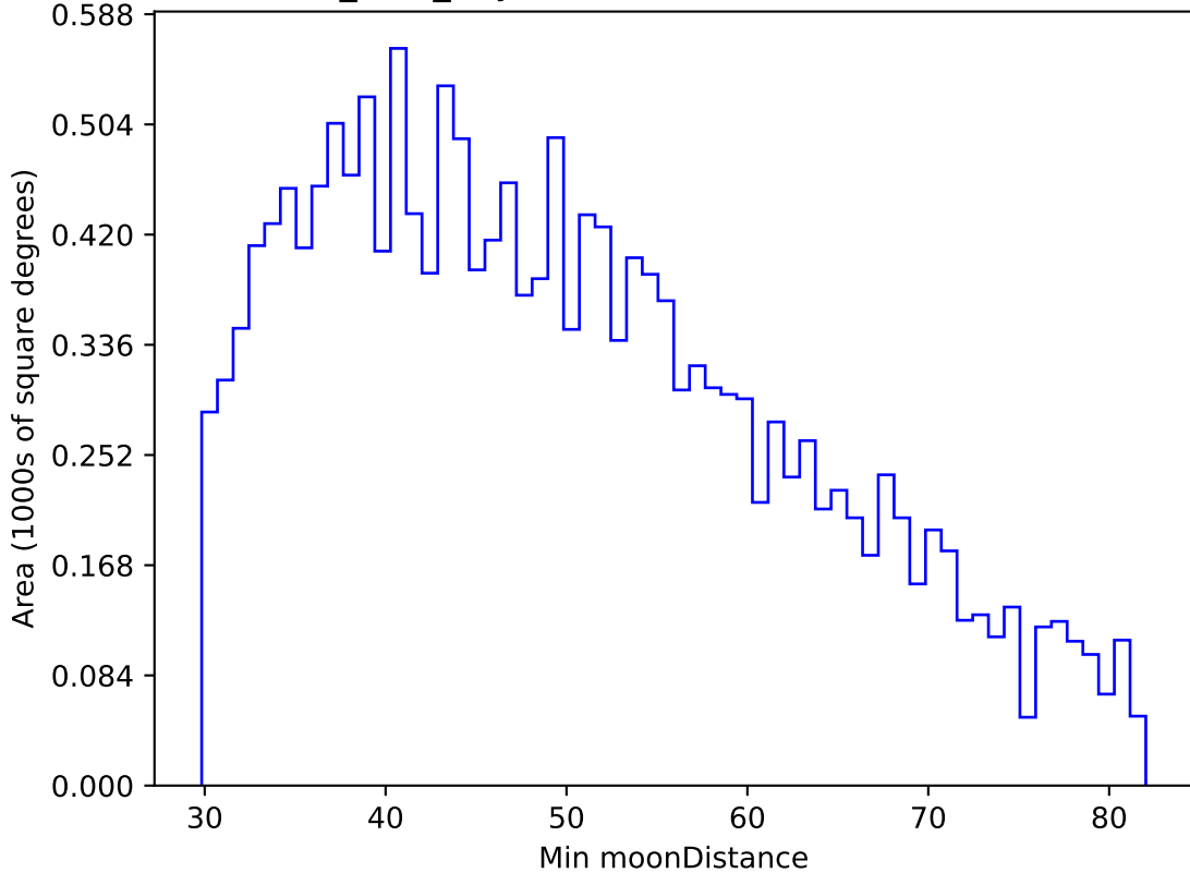
roman_v3.3_10yrs WFD u band: Min moonDistance
