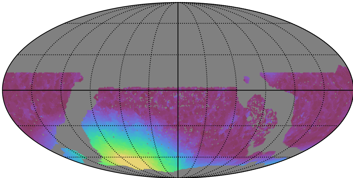
roman_v3.3_10yrs WFD r band: Min moonDistance
