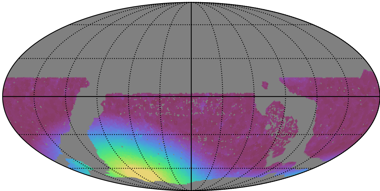
roman_v3.3_10yrs WFD i band: Min moonDistance
