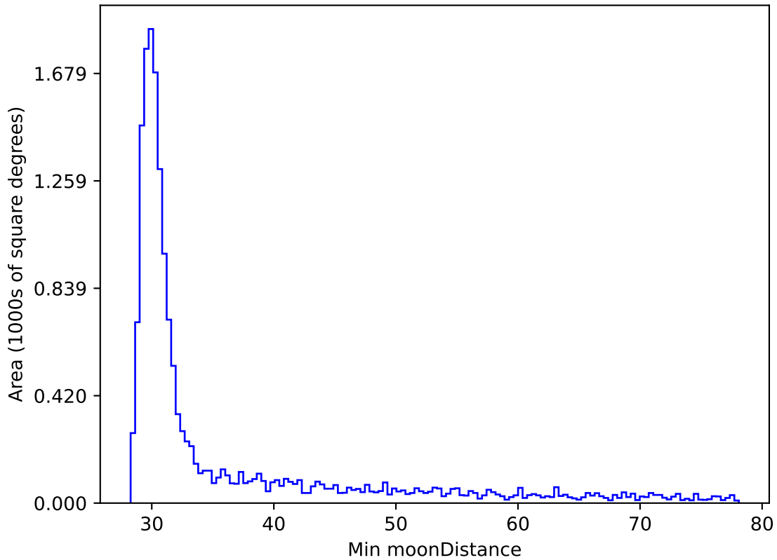
roman_v3.3_10yrs WFD i band: Min moonDistance
