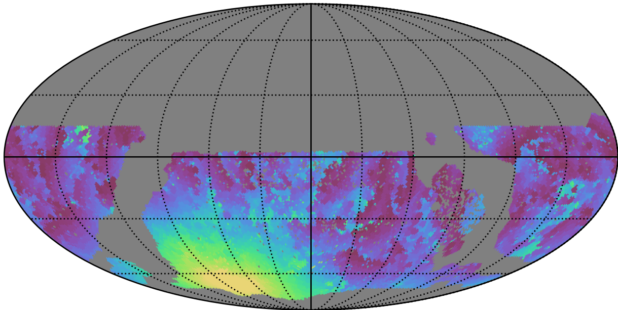
roman_v3.3_10yrs WFD g band: Min moonDistance
