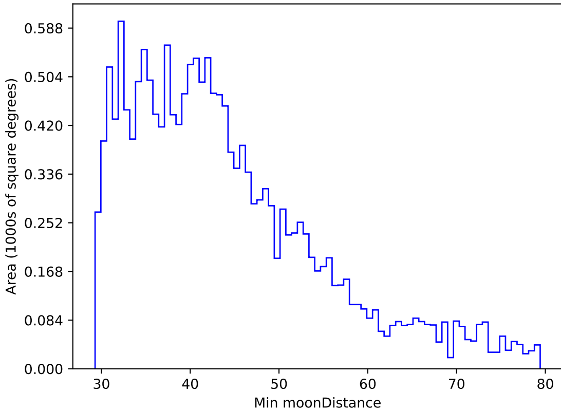
roman_v3.3_10yrs WFD g band: Min moonDistance
