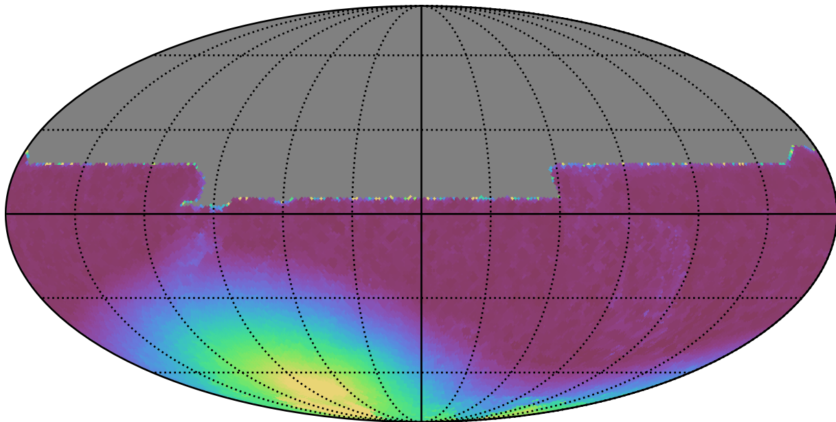
roman_v3.3_10yrs All sky y band: Min moonDistance
