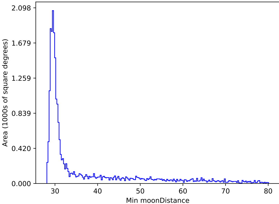
roman_v3.3_10yrs All sky y band: Min moonDistance
