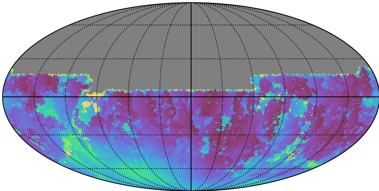
roman_v3.3_10yrs All sky u band: Min moonDistance
