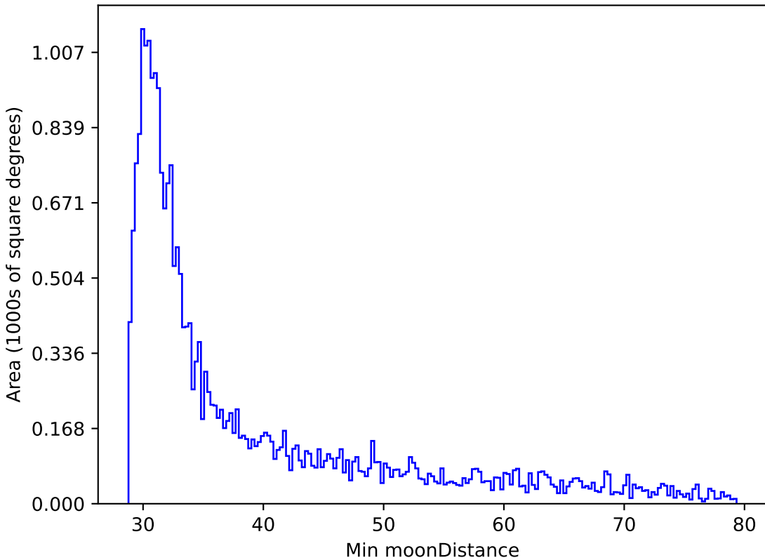
roman_v3.3_10yrs All sky r band: Min moonDistance
