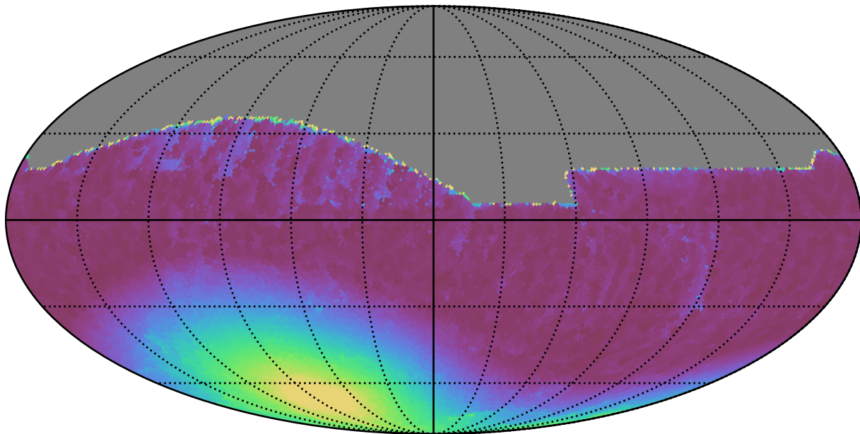
roman_v3.3_10yrs All sky i band: Min moonDistance
