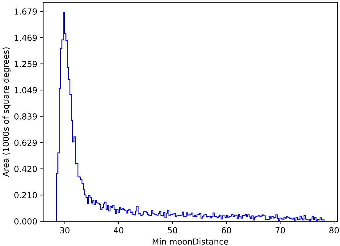
roman_v3.3_10yrs All sky i band: Min moonDistance
