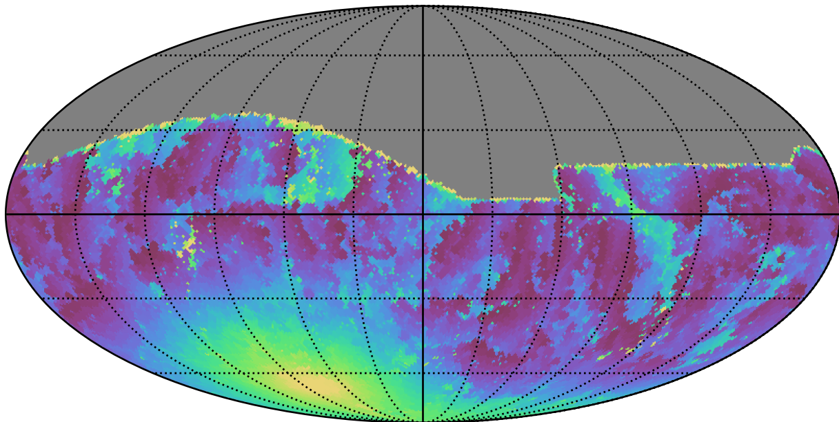
roman_v3.3_10yrs All sky g band: Min moonDistance
