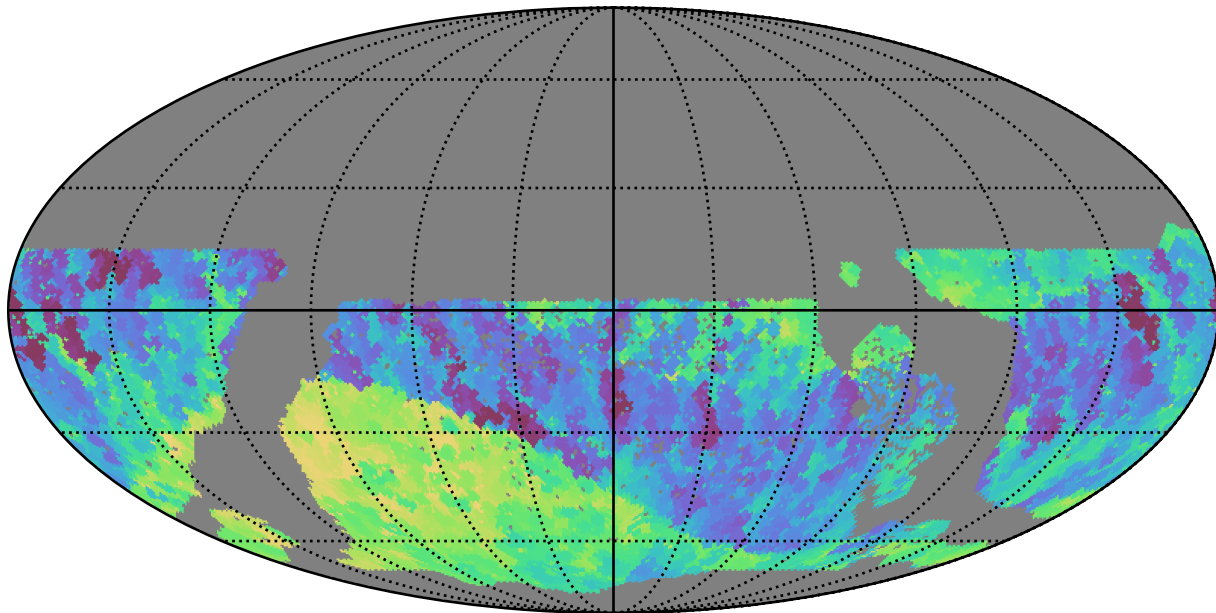
roman_v3.3_10yrs WFD z band: Min fiveSigmaDepth
