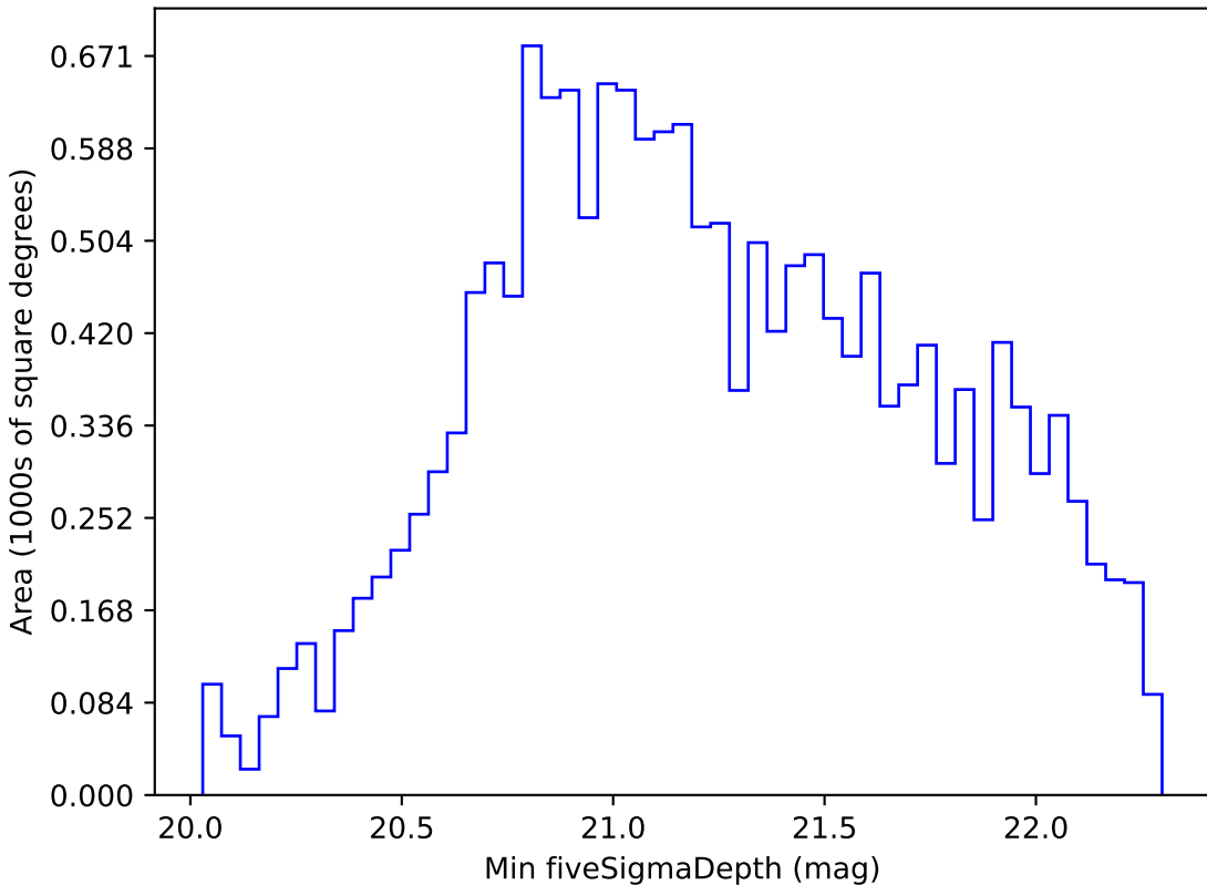
roman_v3.3_10yrs WFD z band: Min fiveSigmaDepth
