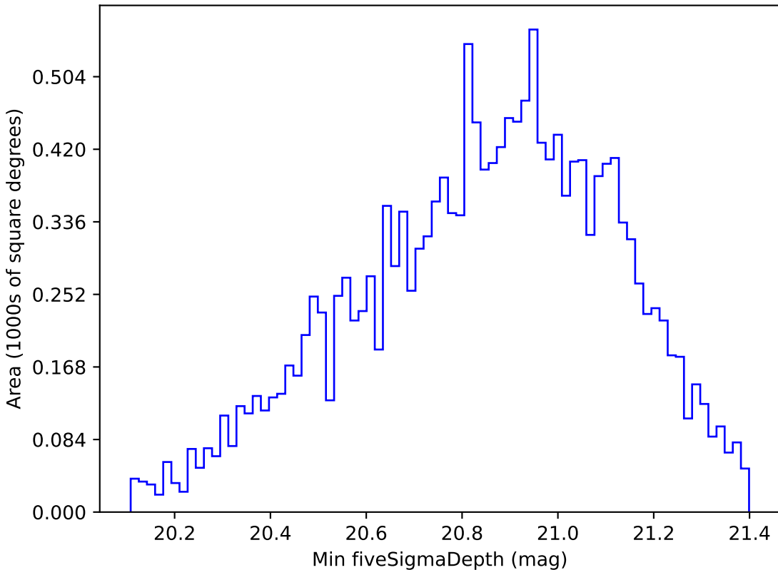
roman_v3.3_10yrs WFD y band: Min fiveSigmaDepth
