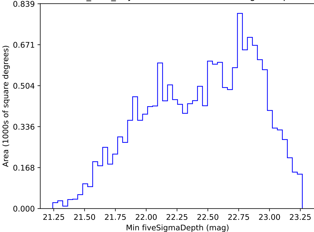
roman_v3.3_10yrs WFD r band: Min fiveSigmaDepth
