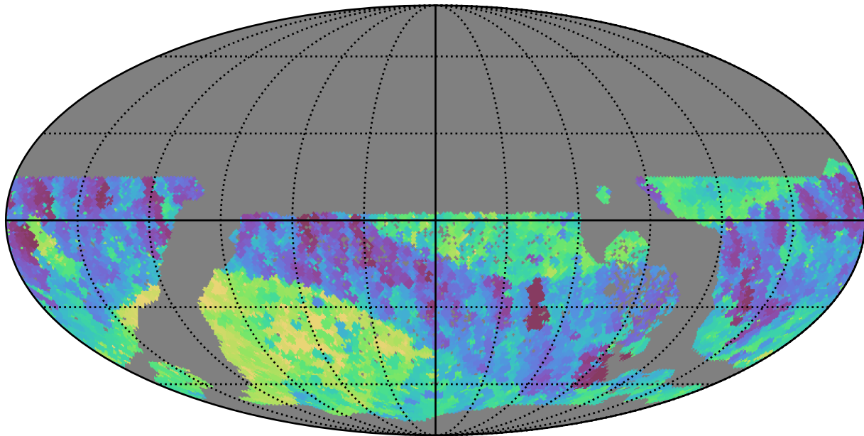
roman_v3.3_10yrs WFD i band: Min fiveSigmaDepth
