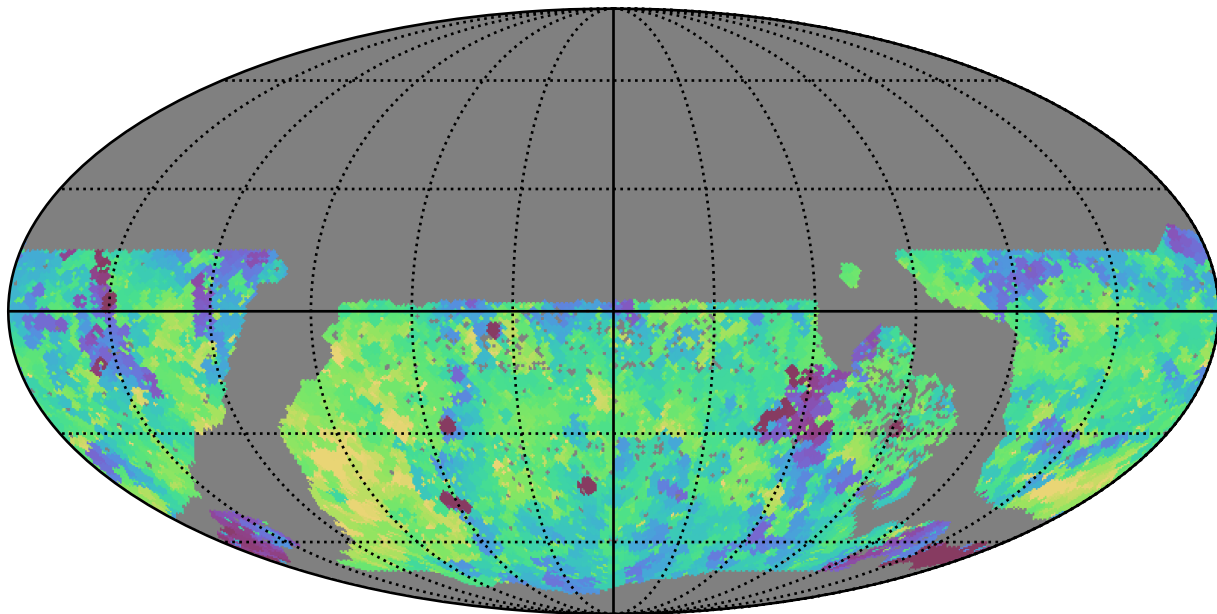
roman_v3.3_10yrs WFD g band: Min fiveSigmaDepth
