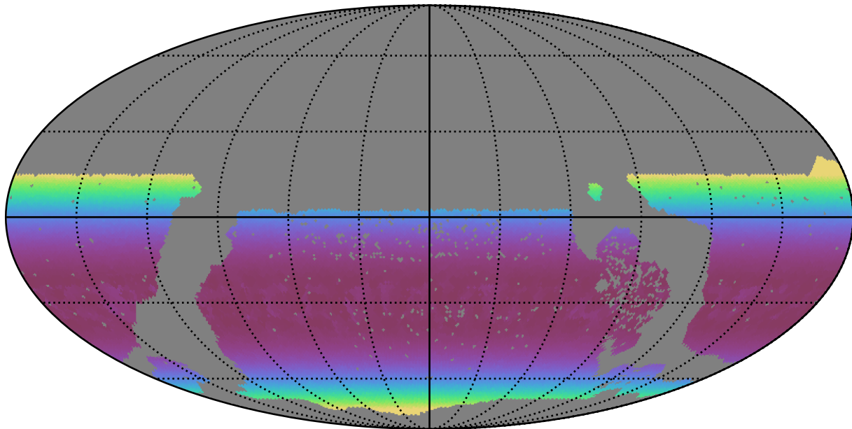
roman_v3.3_10yrs WFD y band: Min airmass
