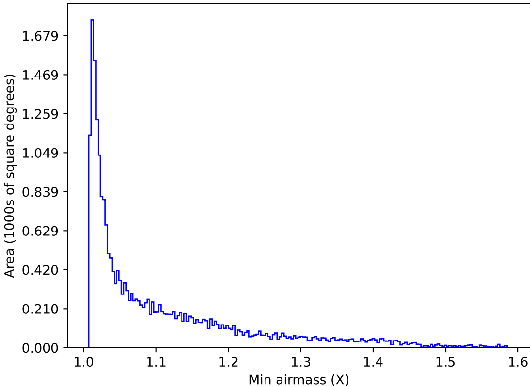
roman_v3.3_10yrs All sky y band: Min airmass
