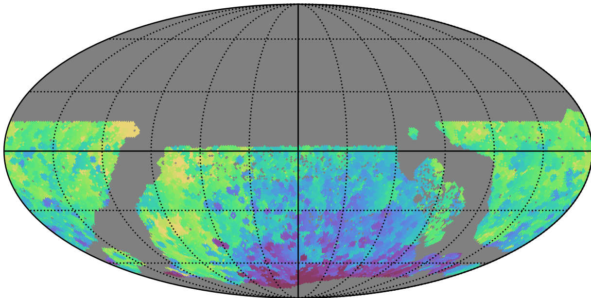
roman_v3.3_10yrs WFD y band: Min HA
