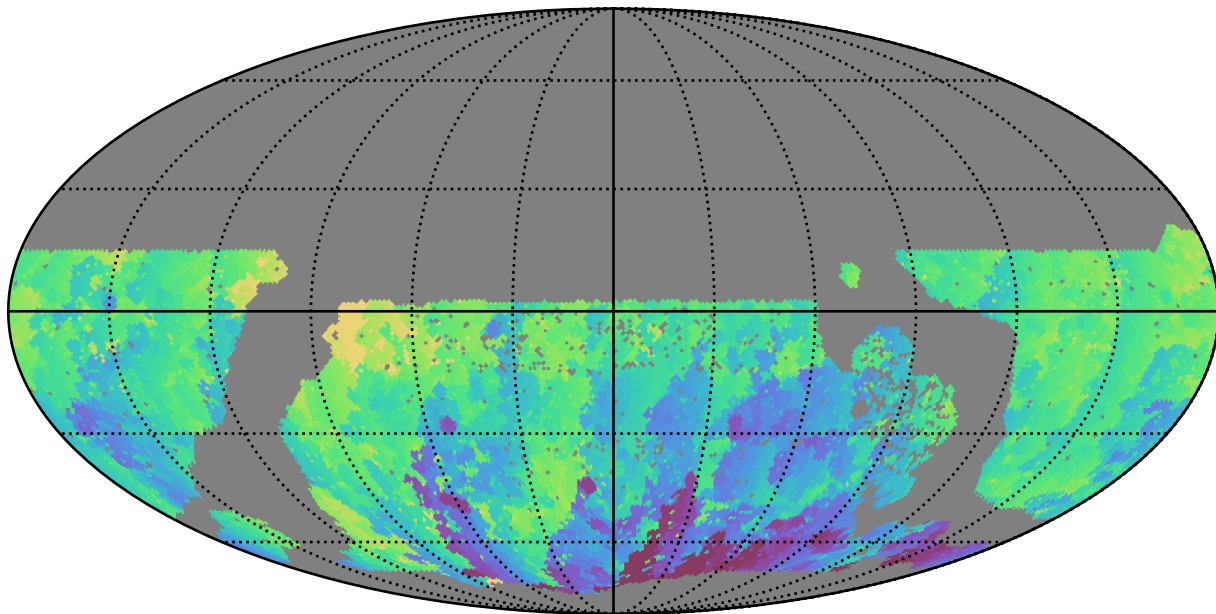
roman_v3.3_10yrs WFD u band: Min HA
