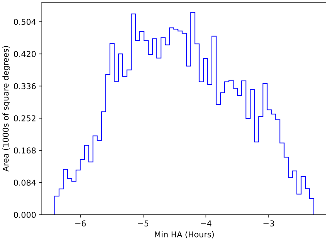
roman_v3.3_10yrs WFD r band: Min HA
