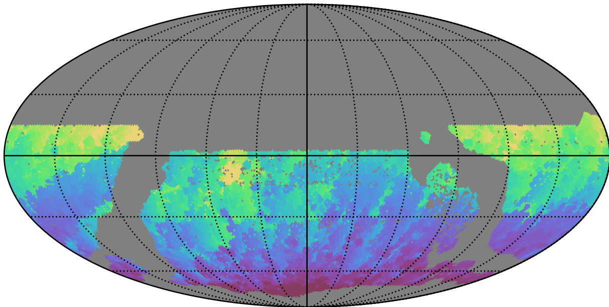
roman_v3.3_10yrs WFD i band: Min HA
