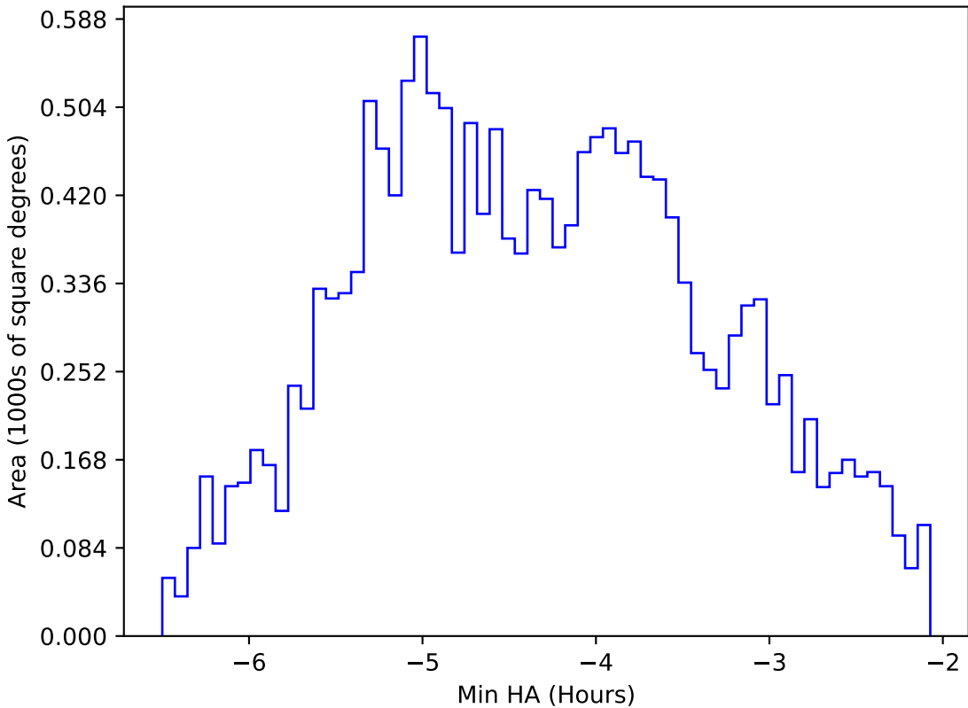
roman_v3.3_10yrs WFD i band: Min HA
