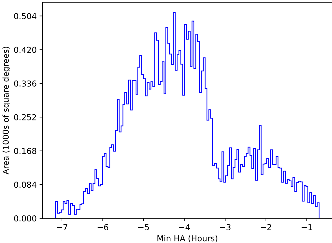
roman_v3.3_10yrs All sky z band: Min HA
