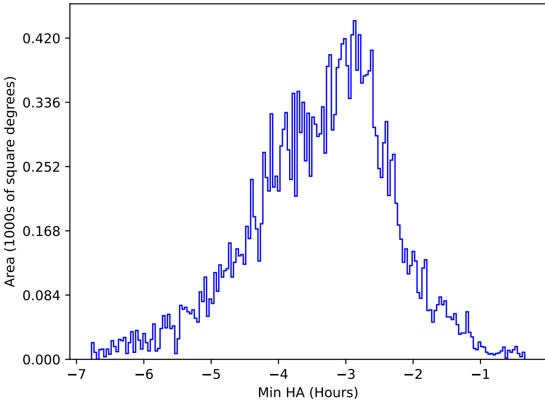
roman_v3.3_10yrs All sky y band: Min HA
