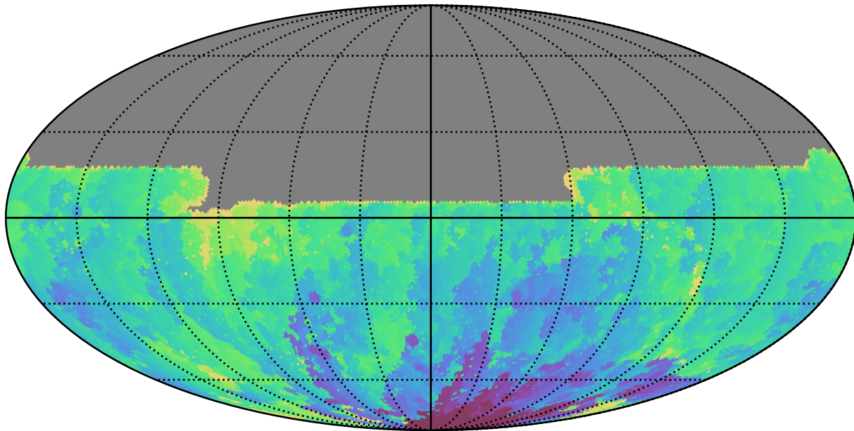
roman_v3.3_10yrs All sky u band: Min HA
