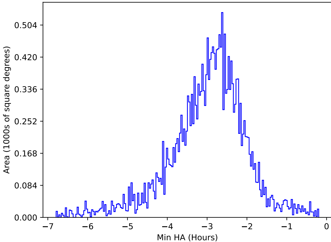
roman_v3.3_10yrs All sky u band: Min HA
