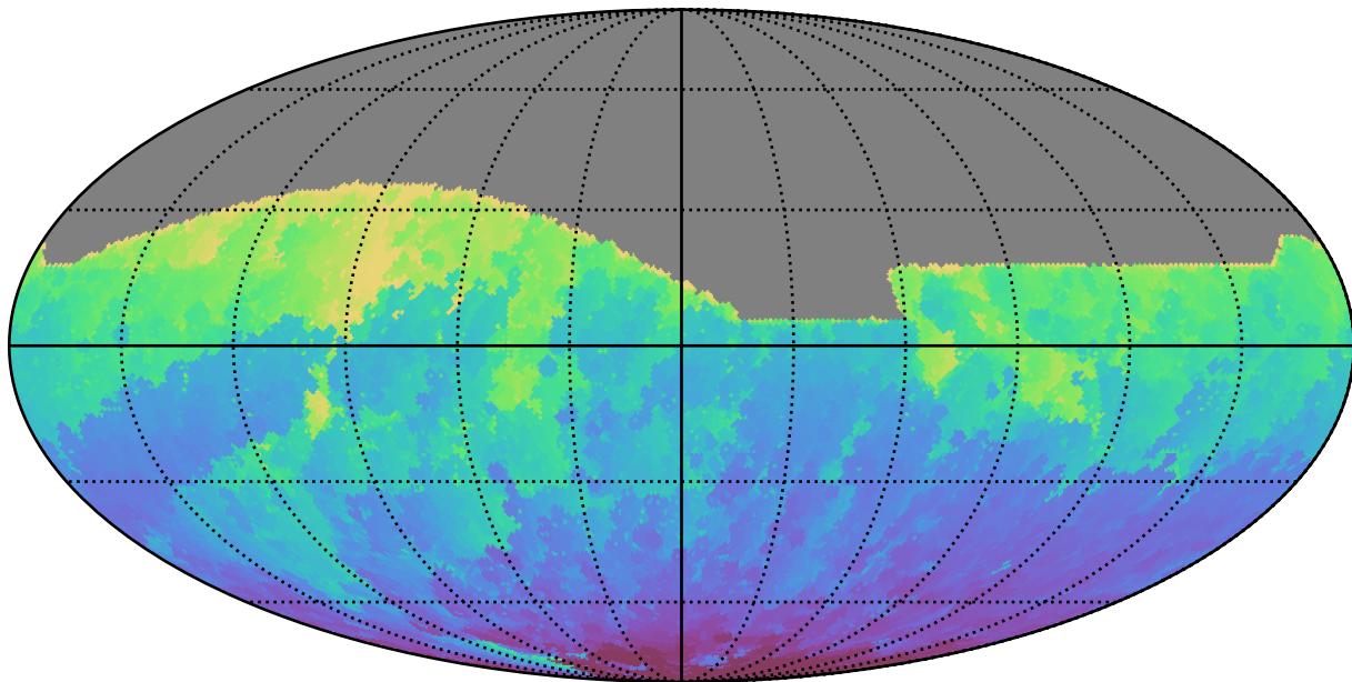
roman_v3.3_10yrs All sky i band: Min HA
