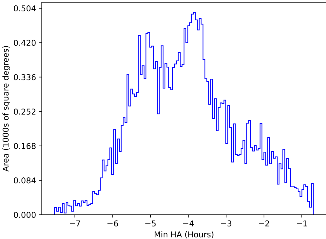
roman_v3.3_10yrs All sky i band: Min HA
