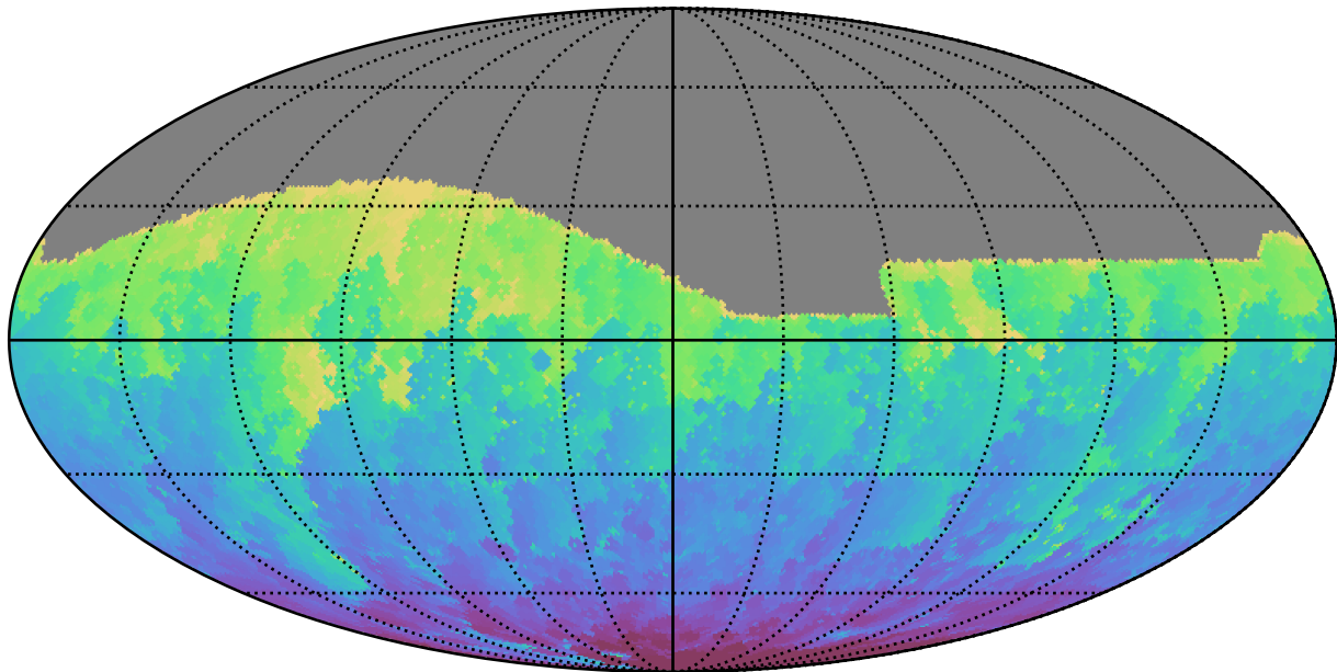
roman_v3.3_10yrs All sky g band: Min HA
