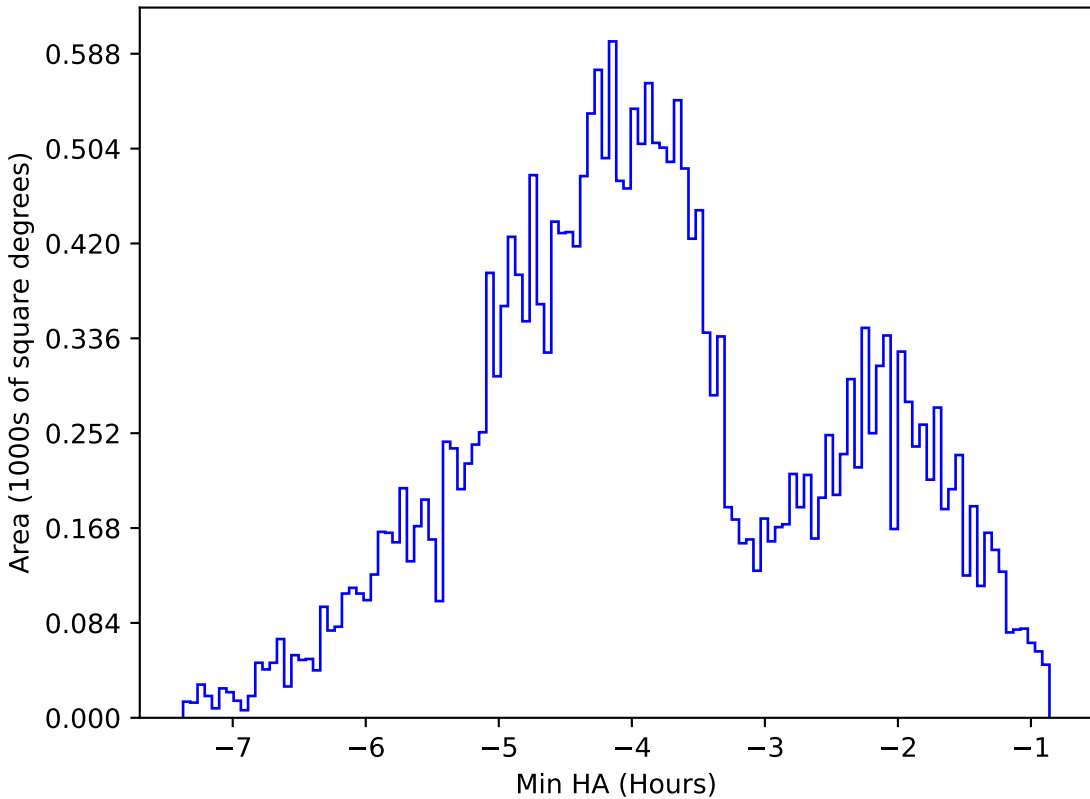
roman_v3.3_10yrs All sky g band: Min HA
