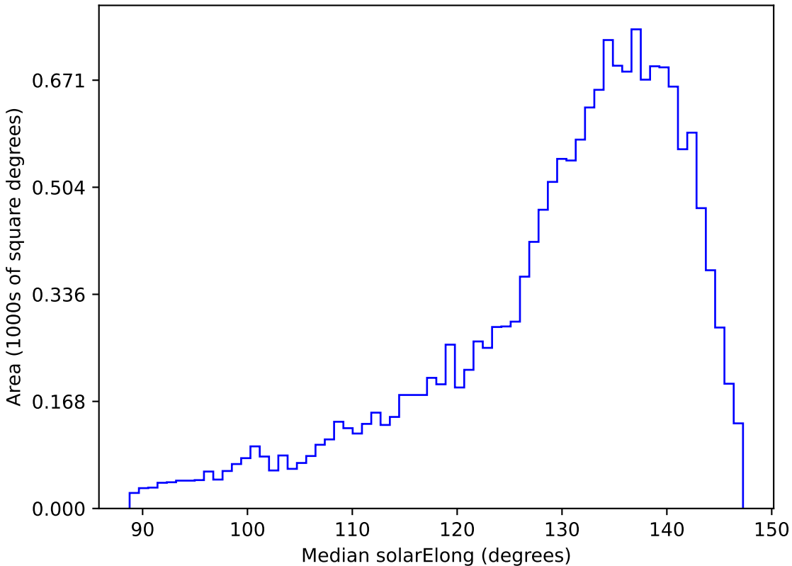
roman_v3.3_10yrs WFD y band: Median solarElong
