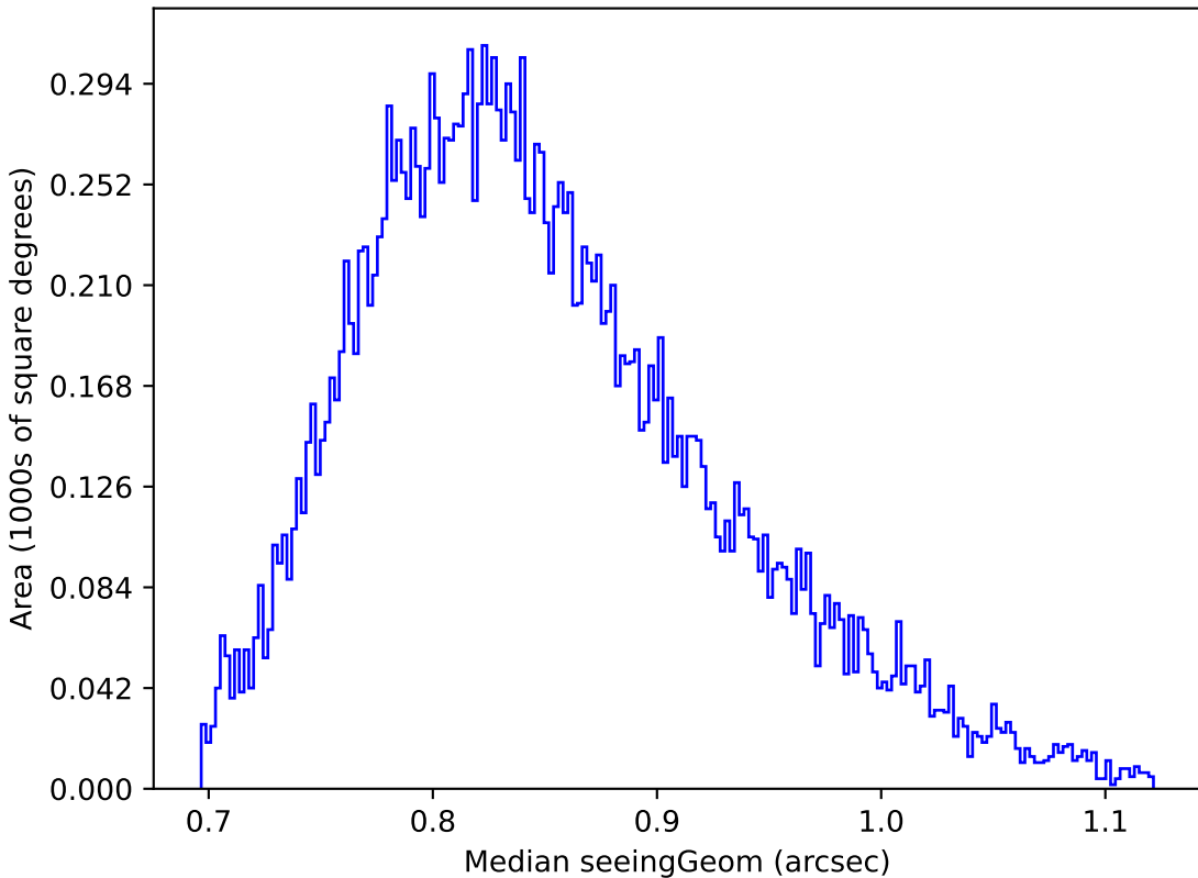
roman_v3.3_10yrs Yr 1 y band: Median seeingGeom
