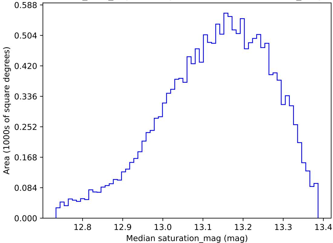
roman_v3.3_10yrs WFD y band: Median saturation_mag
