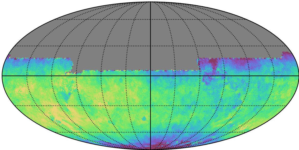
roman_v3.3_10yrs All sky y band: Median saturation_mag
