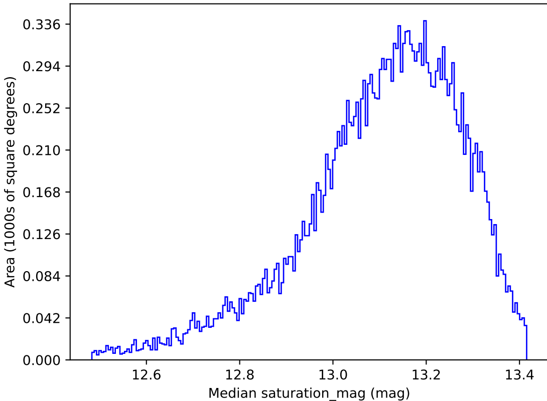
roman_v3.3_10yrs All sky y band: Median saturation_mag
