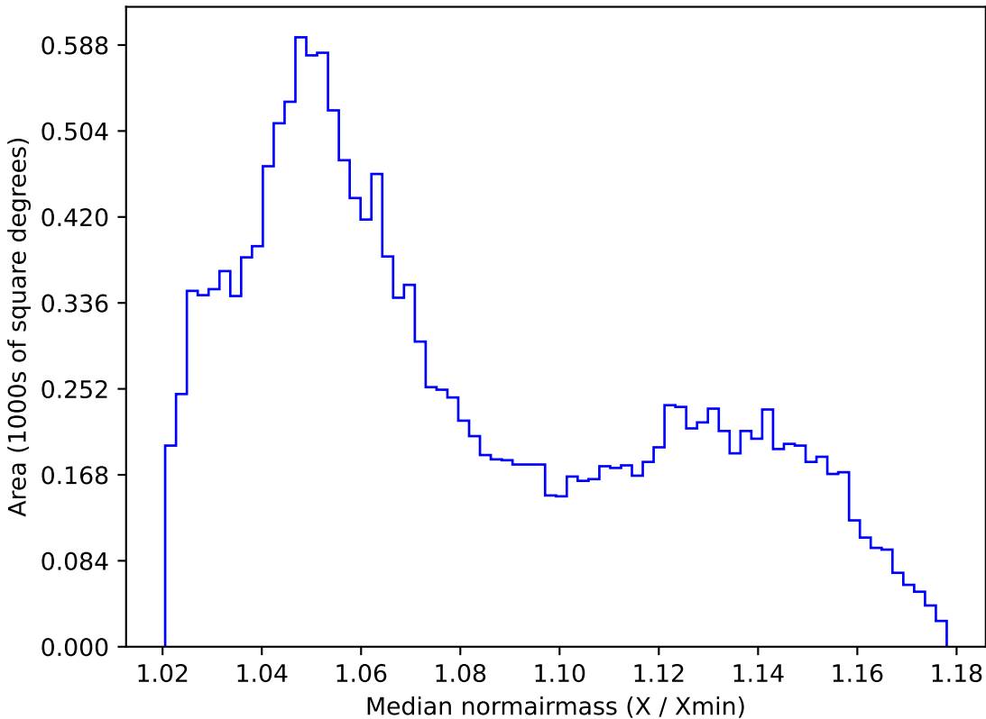
roman_v3.3_10yrs WFD z band: Median normairmass
