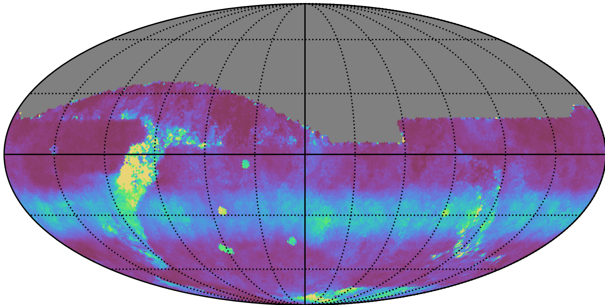
roman_v3.3_10yrs All sky z band: Median normairmass
