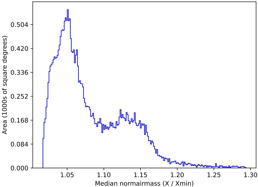
roman_v3.3_10yrs All sky z band: Median normairmass
