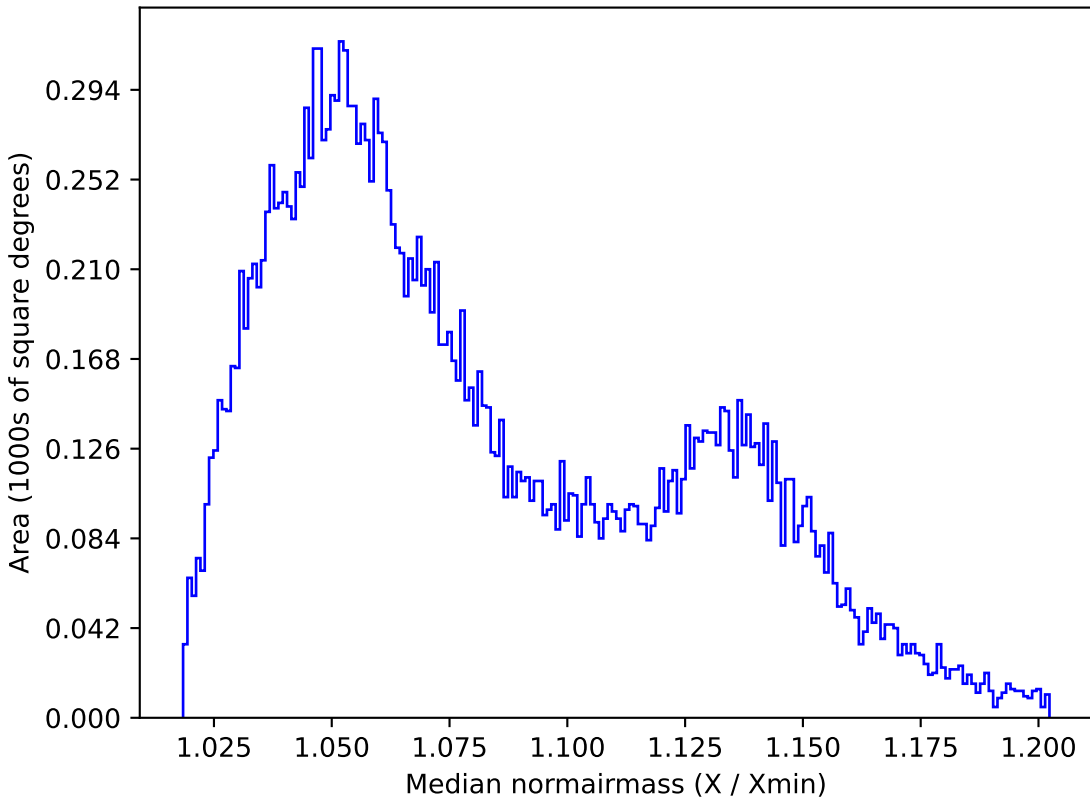
roman_v3.3_10yrs All sky y band: Median normairmass
