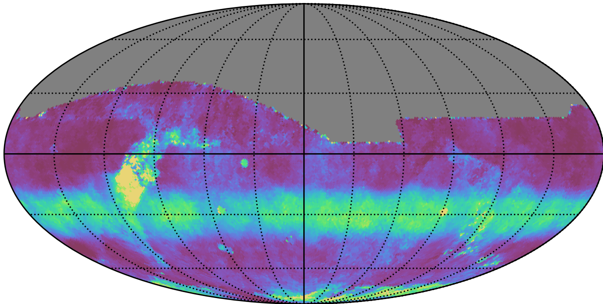
roman_v3.3_10yrs All sky i band: Median normairmass
