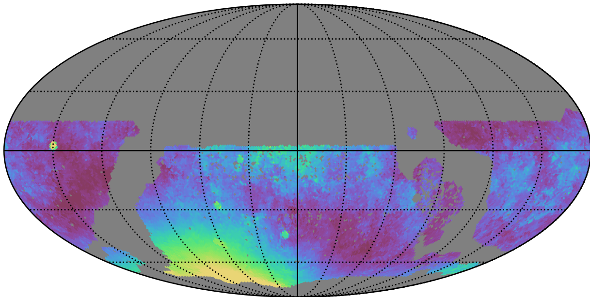
roman_v3.3_10yrs WFD y band: Median moonDistance
