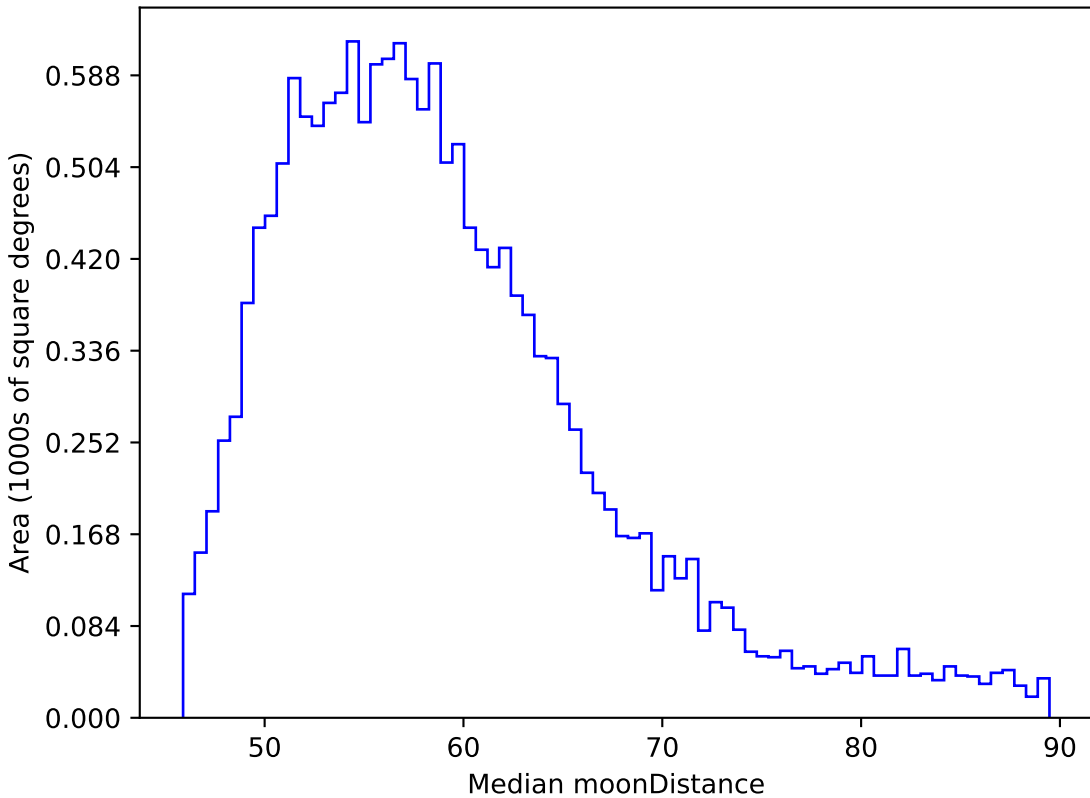
roman_v3.3_10yrs WFD y band: Median moonDistance
