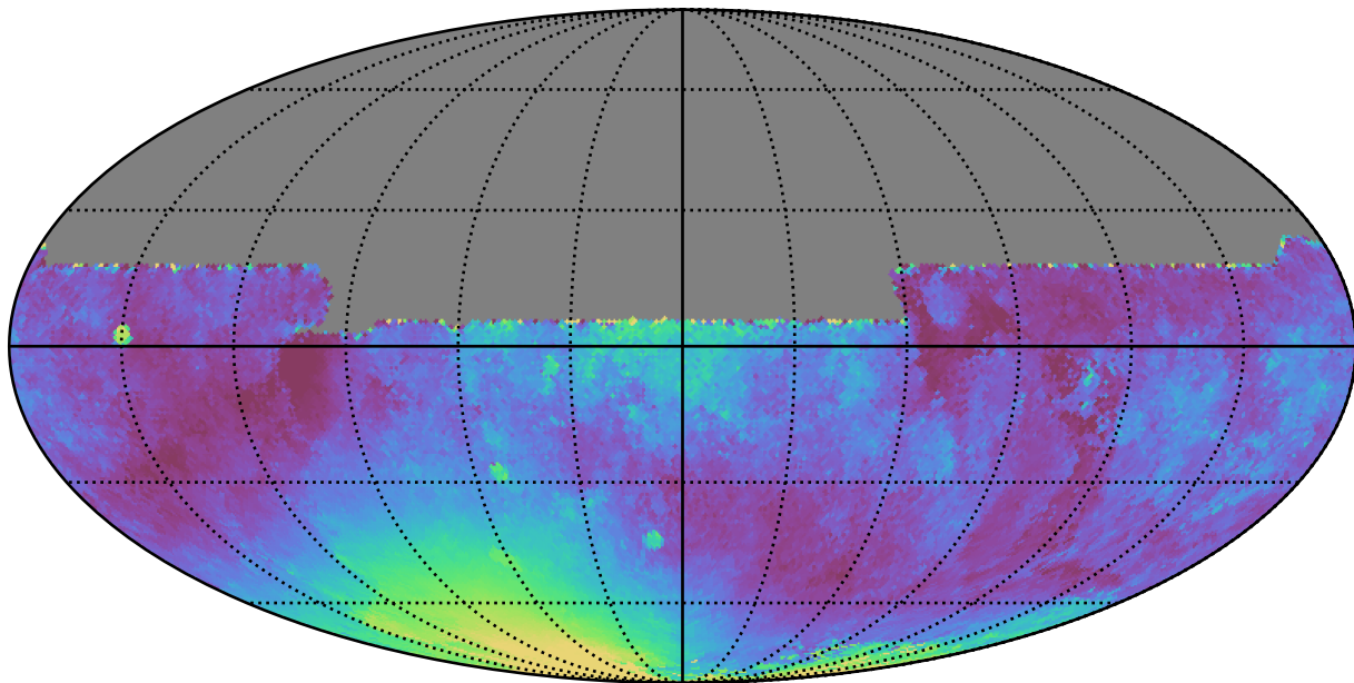
roman_v3.3_10yrs All sky y band: Median moonDistance
