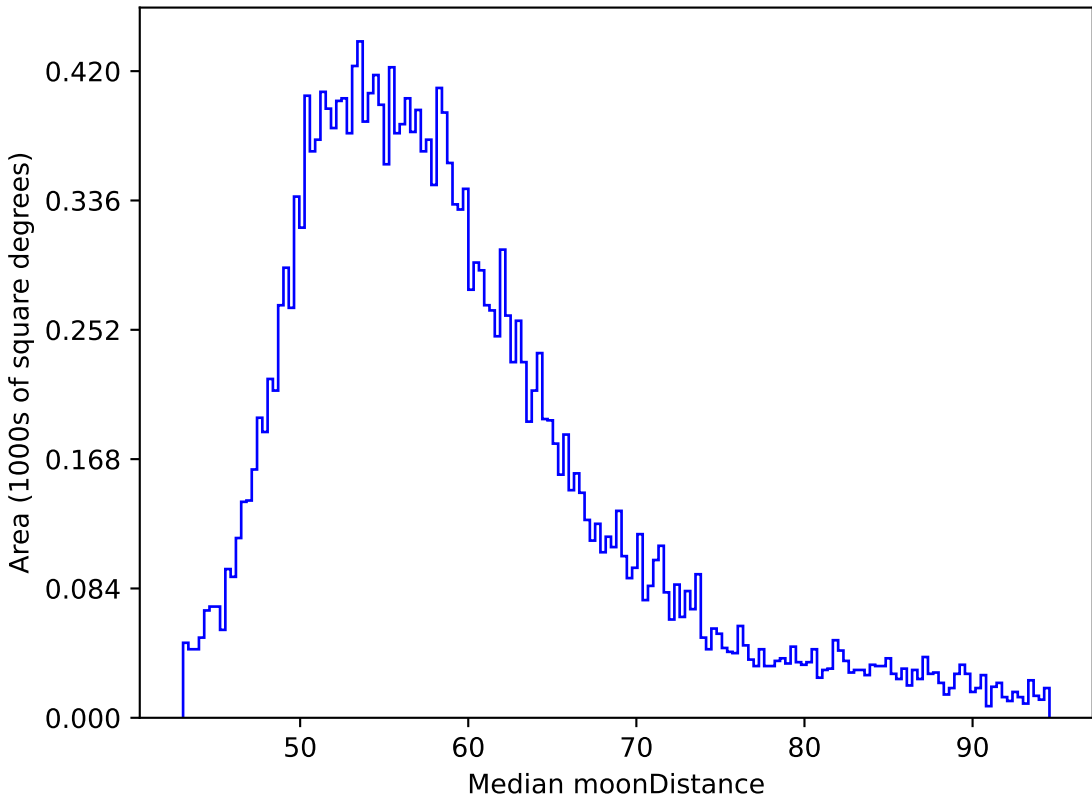
roman_v3.3_10yrs All sky y band: Median moonDistance
