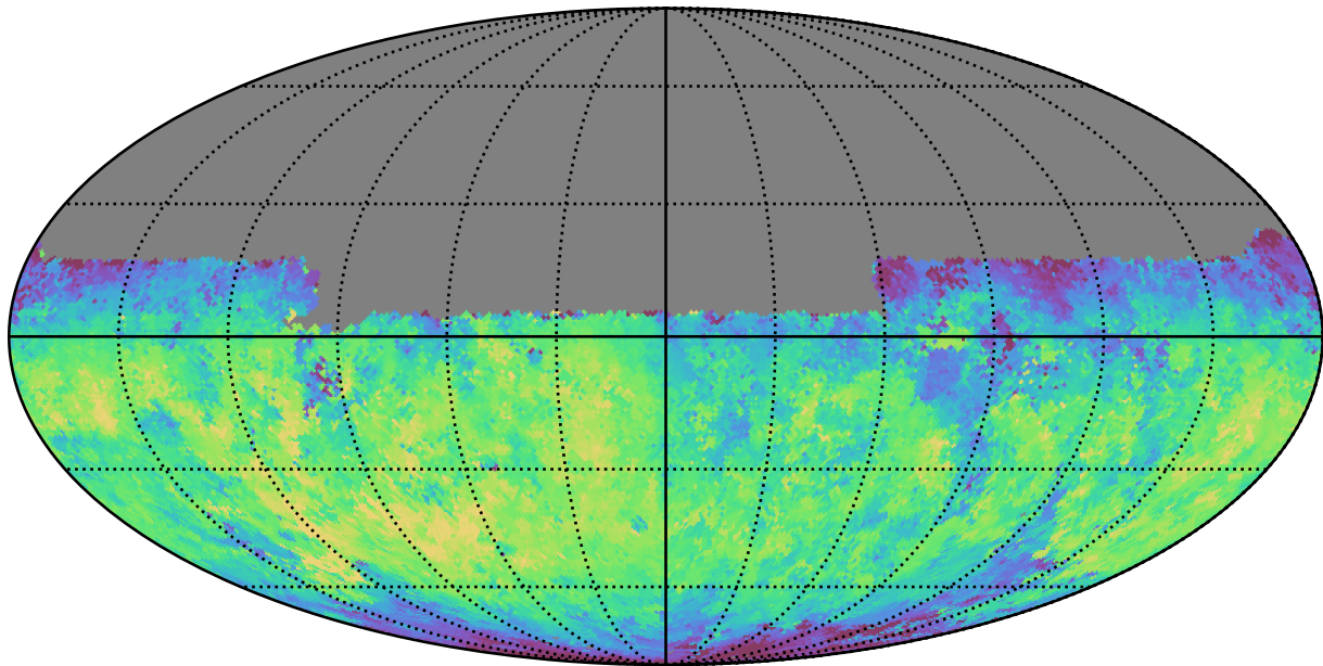
roman_v3.3_10yrs Yr 1 y band: Median fiveSigmaDepth
