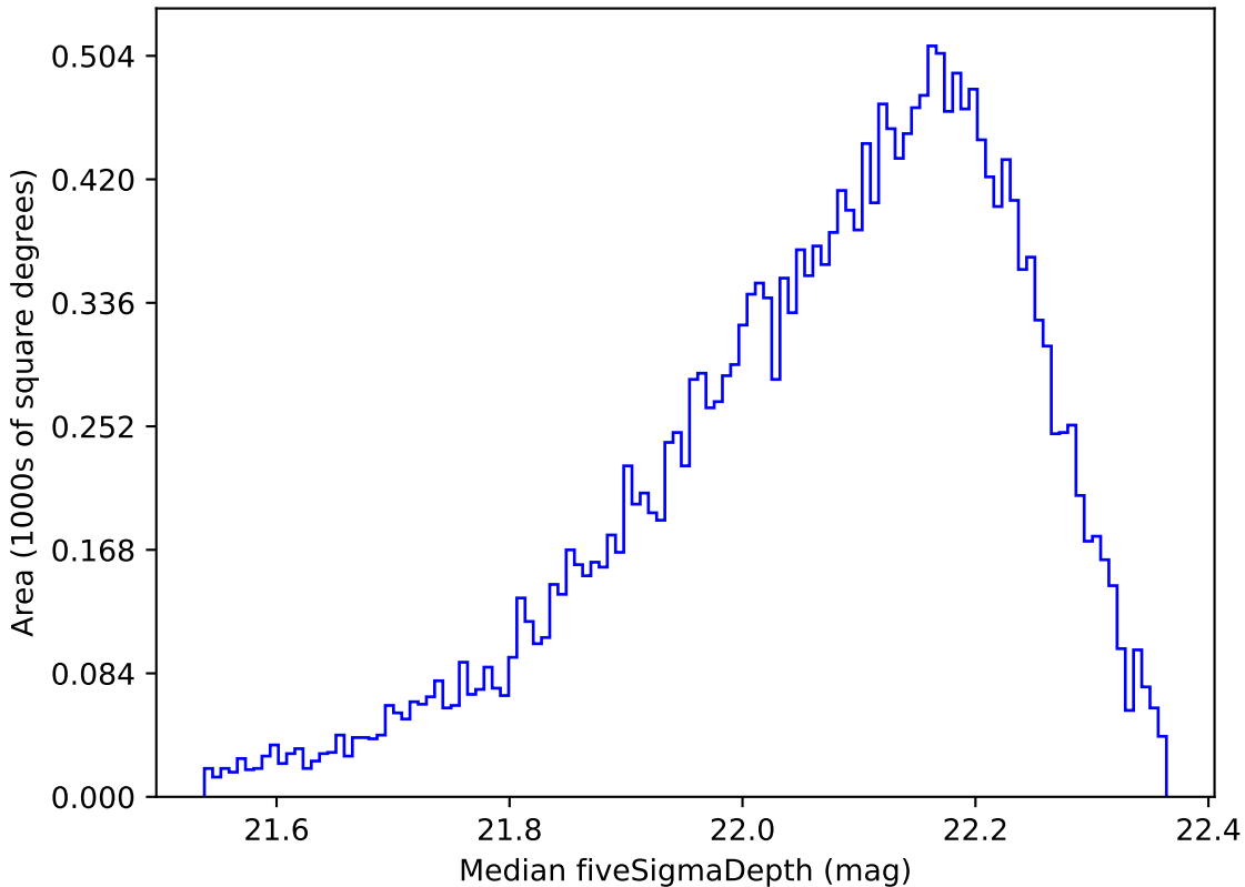
roman_v3.3_10yrs Yr 1 y band: Median fiveSigmaDepth
